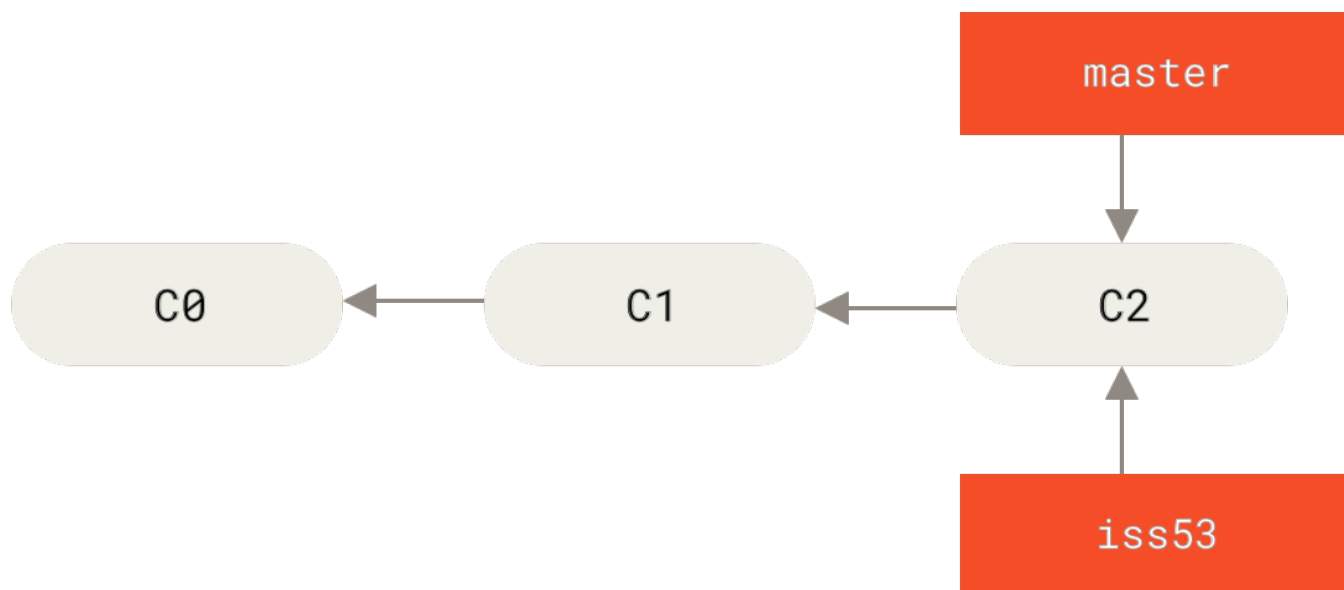
Figure 19. 创建一个新分支指针
