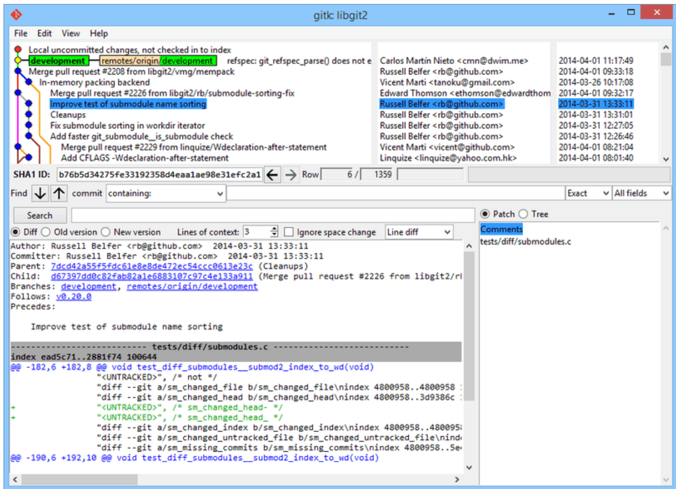
Figure 152. gitk 历史查看器。
