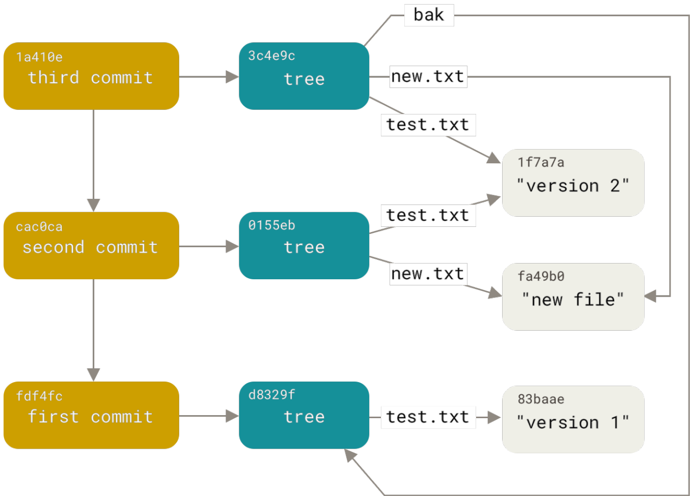
Figure 150. 你的 Git 目录下所有可达的对象。
