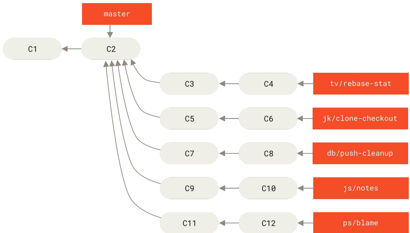
Figure 78. 管理复杂的一系列接收贡献的平行主题分支。
