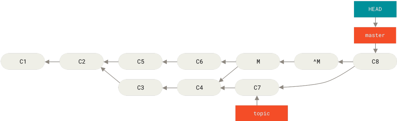
Figure 141. 含有坏掉合并的历史
