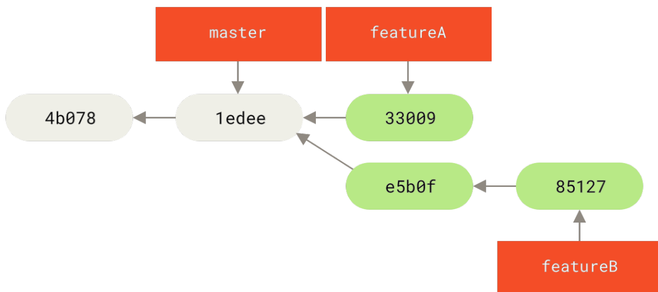
Figure 66. Jessica 的初始提交历史
