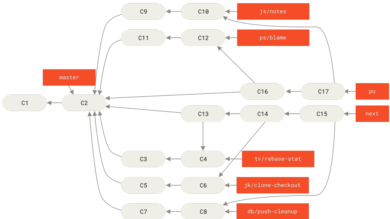
Figure 79. 将贡献的主题分支并入长期整合分支。
