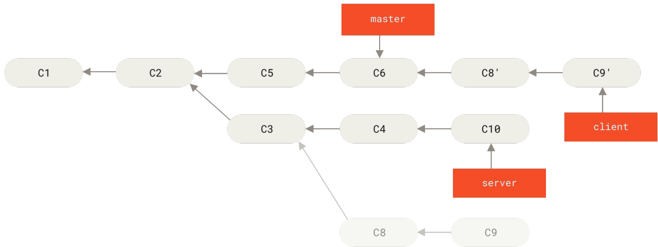
Figure 40. 截取主题分支上的另一个主题分支，然后变基到其他分支
