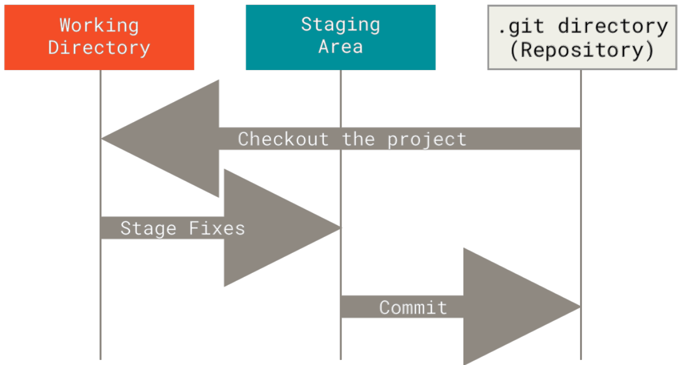
Figure 6. 工作目录、暂存区域以及 Git 仓库。
