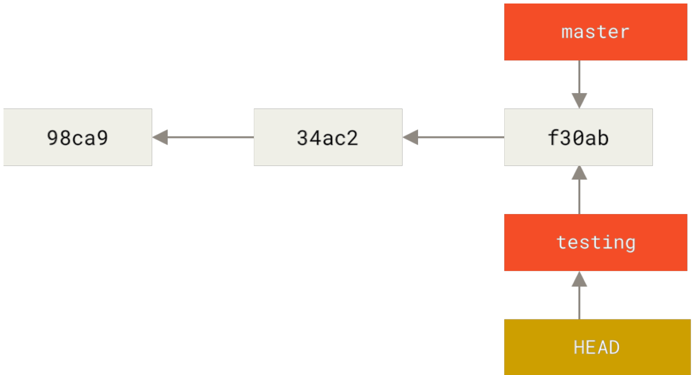
Figure 14. HEAD 指向当前所在的分支
