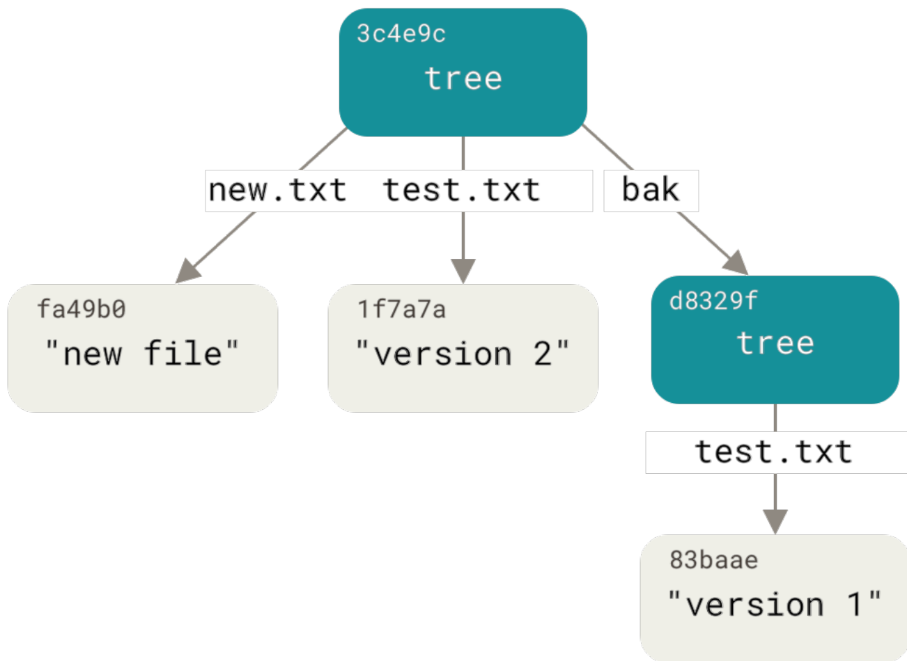
Figure 149. 当前 Git 的数据内容结构。
