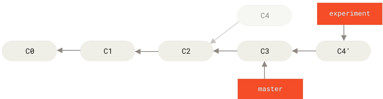
Figure 37. 将 C4 中的修改变基到 C3 上
