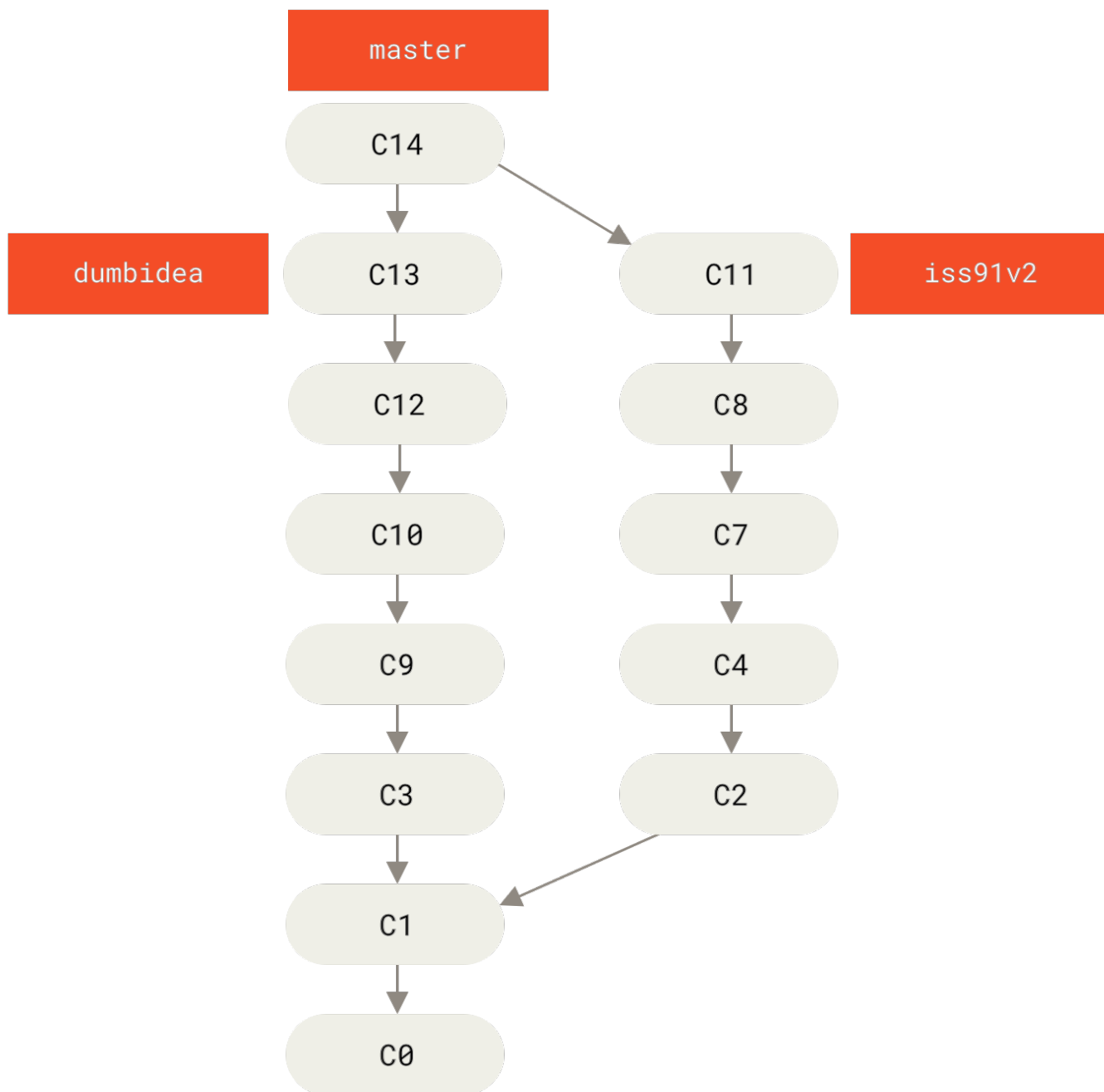
Figure 29. 合并了 dumbidea 和 iss91v2 分支之后的提交历史
