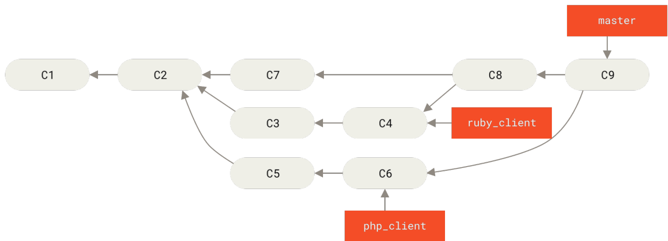
Figure 74. 合并主题分支之后。
