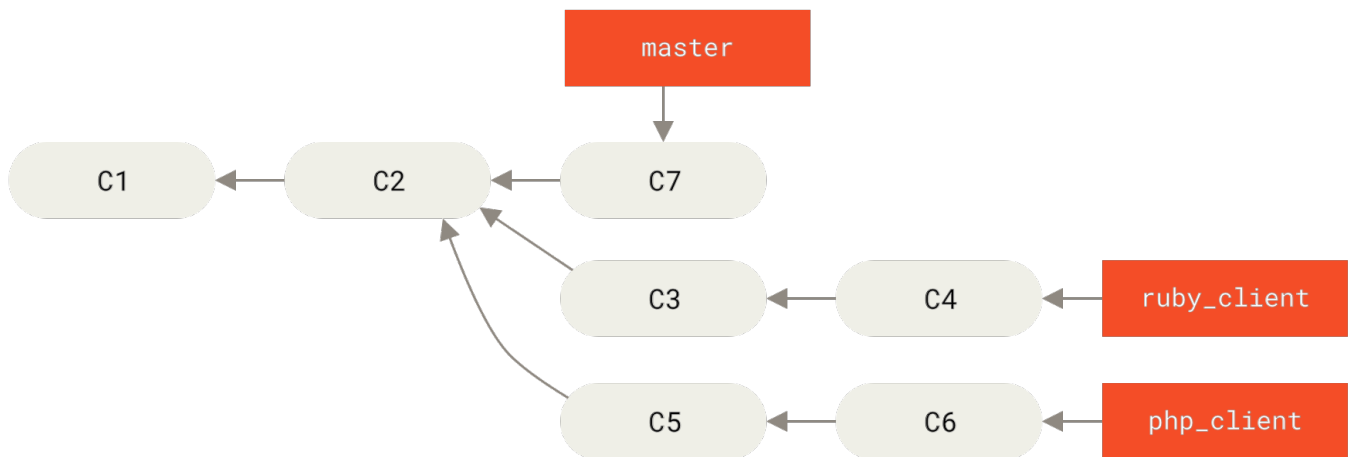
Figure 73. 包含若干主题分支的提交历史。
