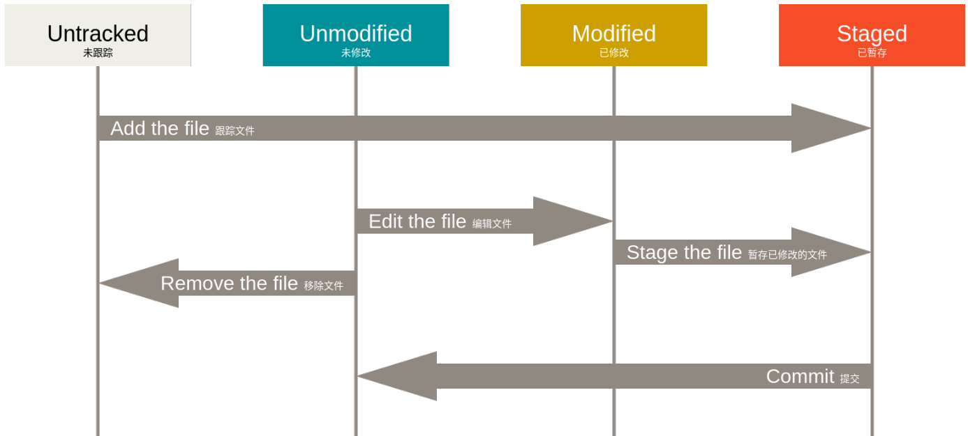
Figure 8. 文件的状态变化周期
