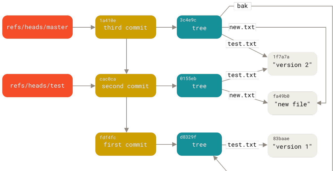
Figure 151. 包含分支引用的 Git 目录对象。
