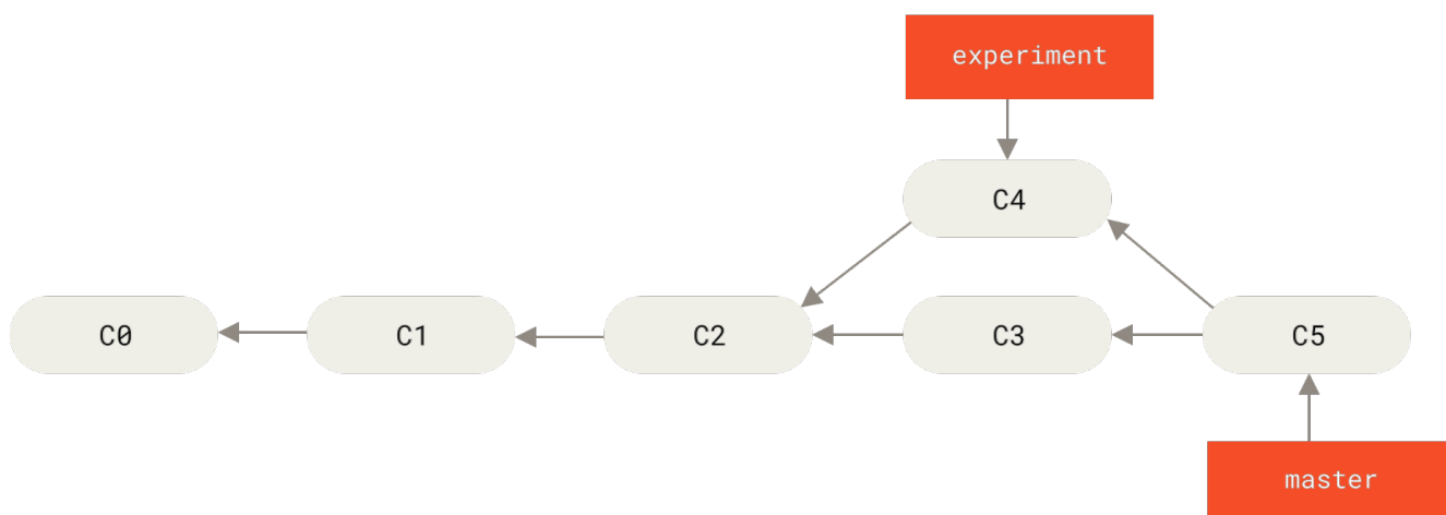
Figure 36. 通过合并操作来整合分叉的历史
