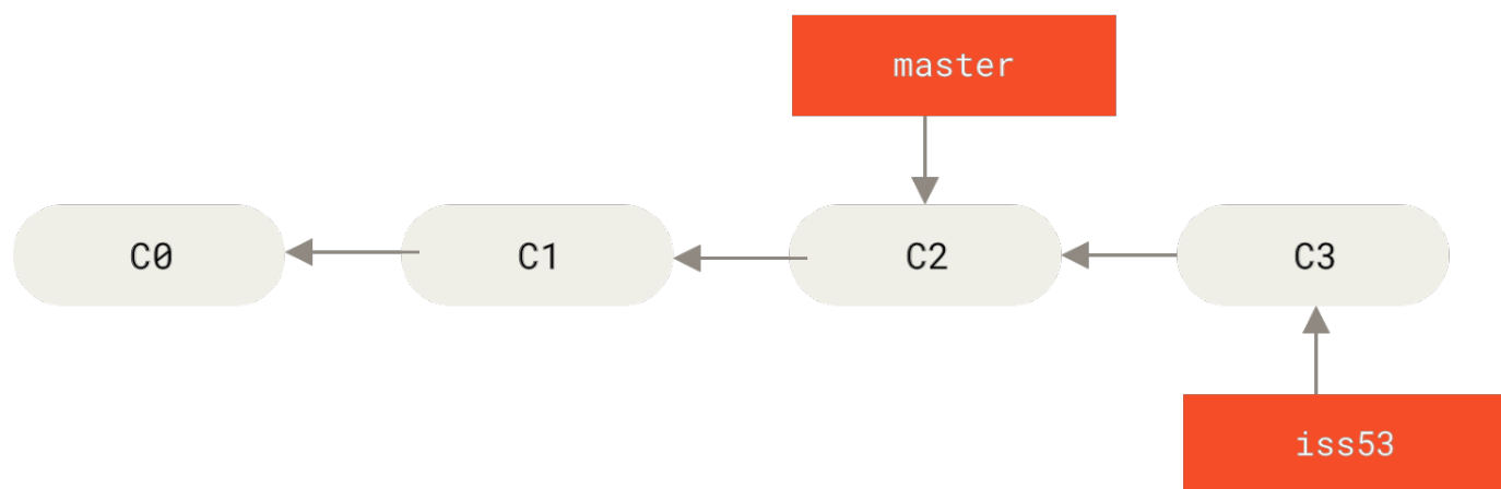
Figure 20. iss53 分支随着工作的进展向前推进
