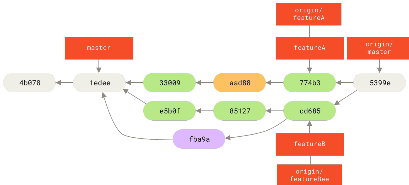
Figure 68. 合并了 Jessica 的两个主题分支后她的历史
