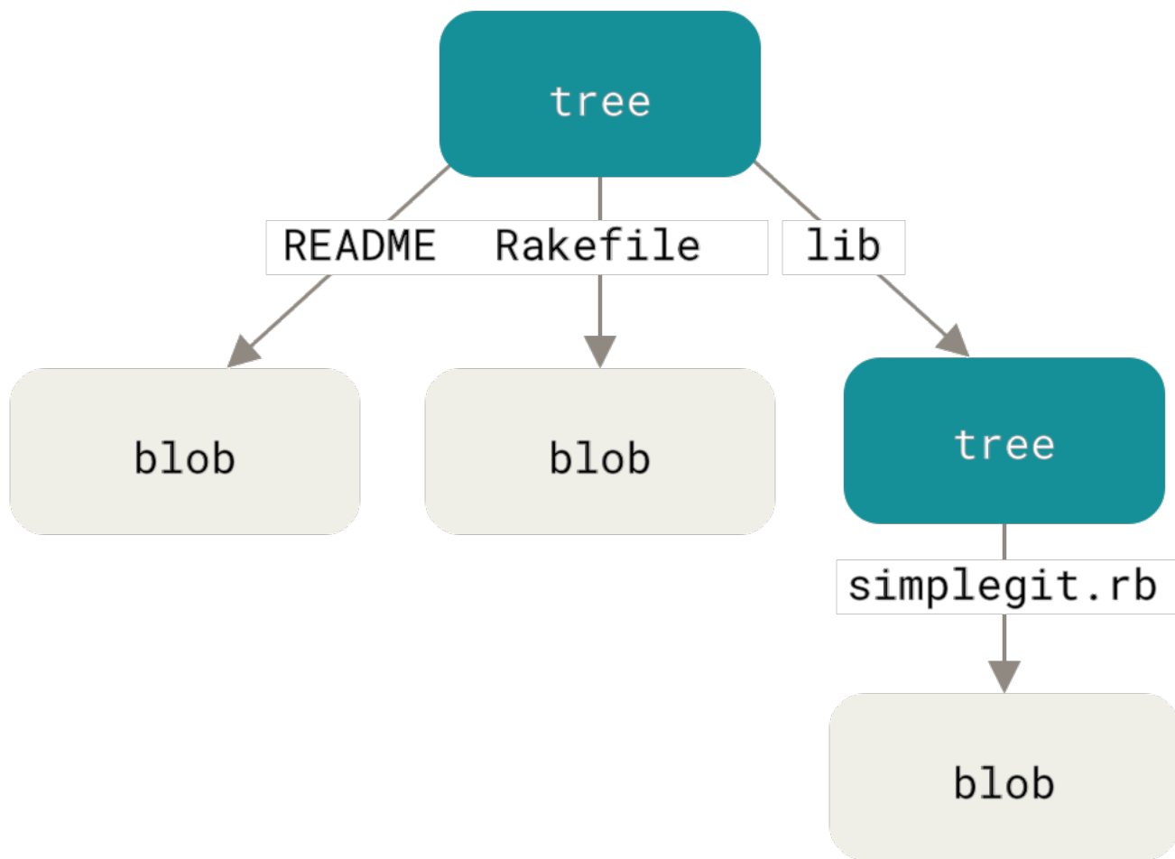
Figure 148. 简化版的 Git 数据模型。
