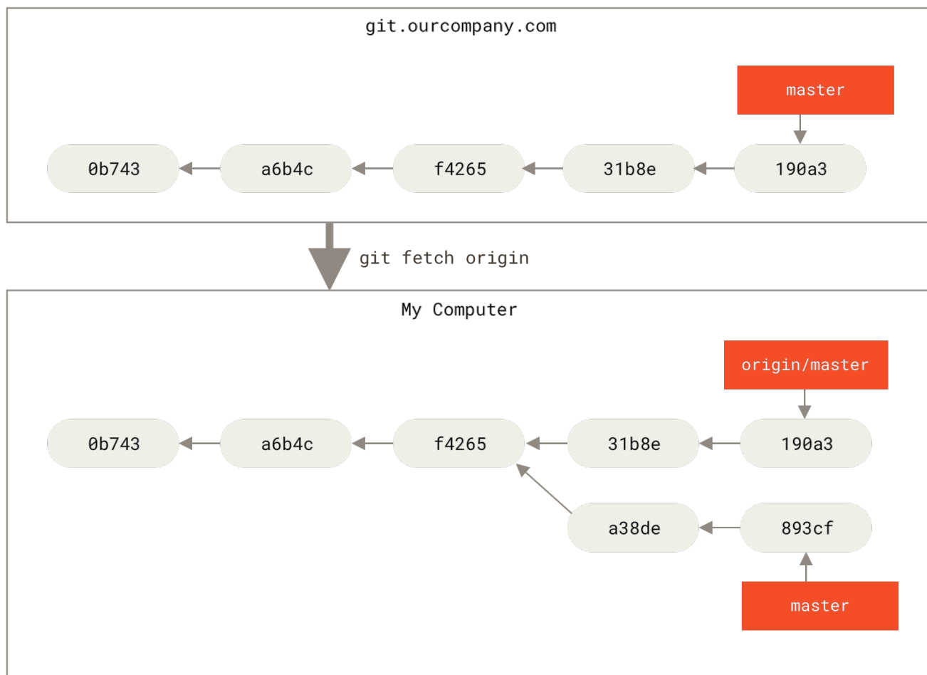
Figure 32. git fetch 更新你的远程跟踪分支
