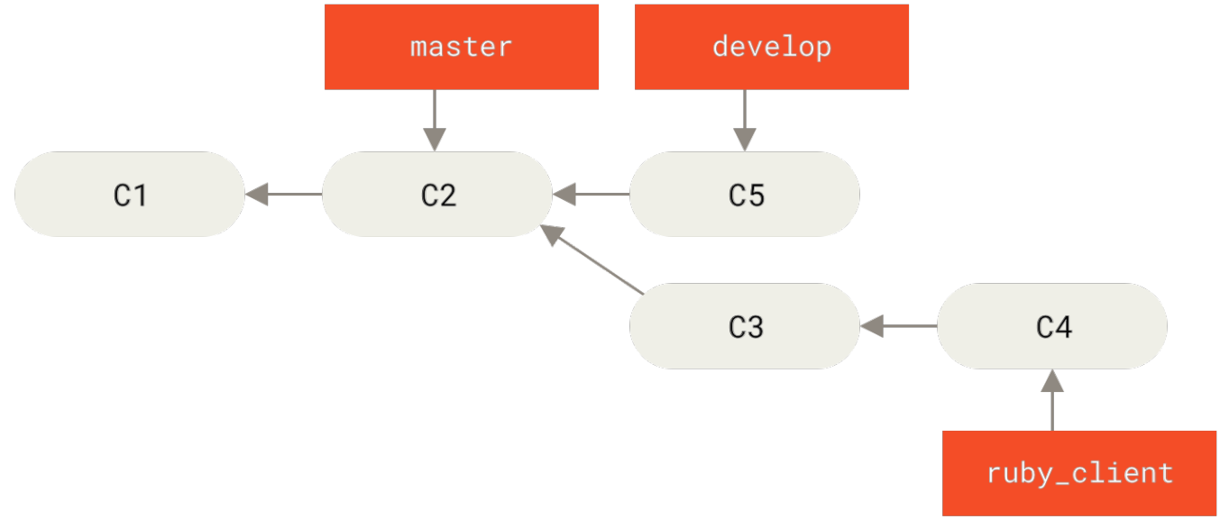
Figure 75. 合并主题分支前。
