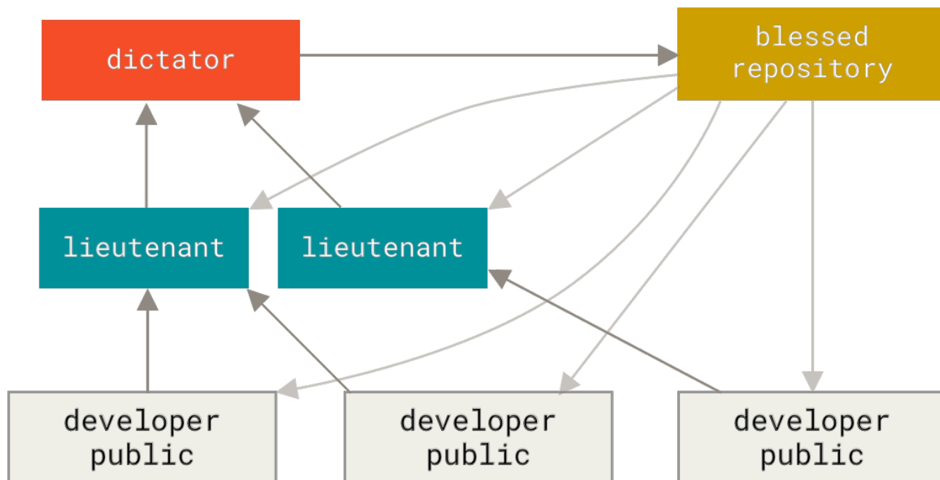
Figure 56. 主管与副主管工作流。
