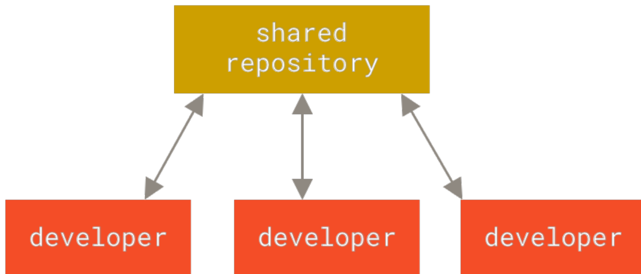
Figure 2. 集中化的版本控制.
