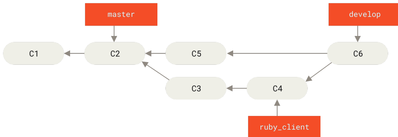
Figure 76. 合并主题分支后。
