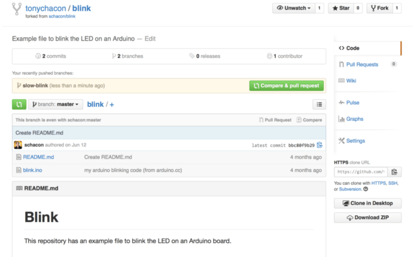
Figure 91. 拉取请求按钮
