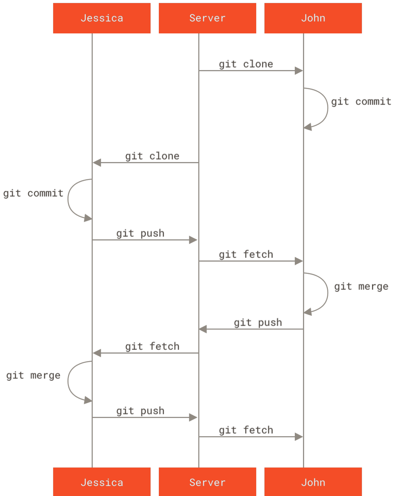
Figure 65. 一个简单的多人 Git 工作流程的通常事件顺序
