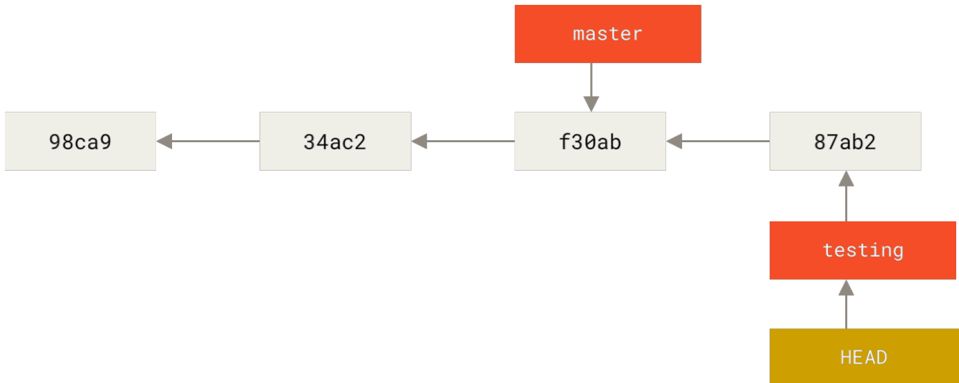
Figure 15. HEAD 分支随着提交操作自动向前移动
